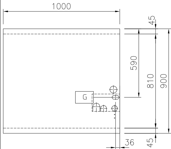
俯视
